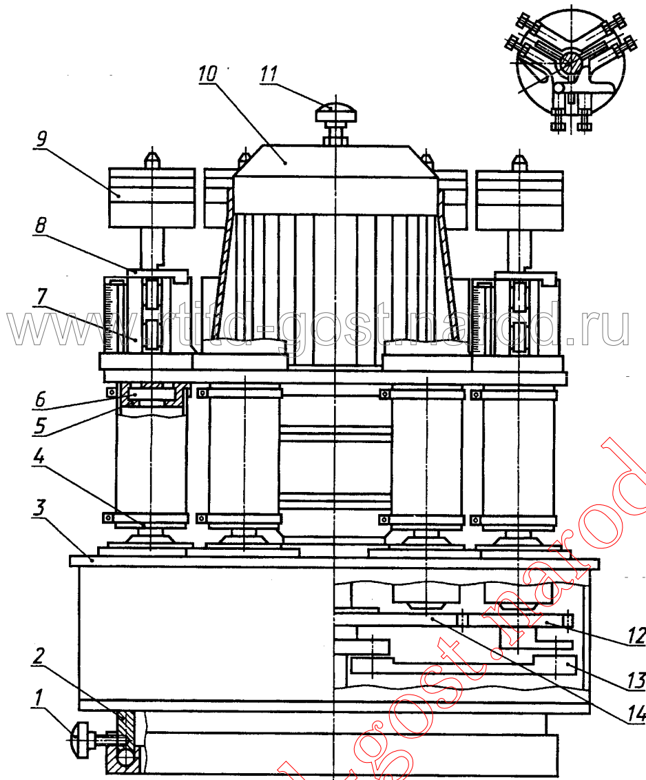
1 — стопорный винт; 2 — опора на шариках; 3 — основание; 4 — нижний зажим; 5 — верхний зажим; 6 — хомут; 7 — направляющий корпус с подшипником; 8 — фиксатор; 9 — съемный груз; 10 — мотор-редуктор; 11 — маховичок; 12 — шестерня; 13 — шатун; 14 — шестерня
