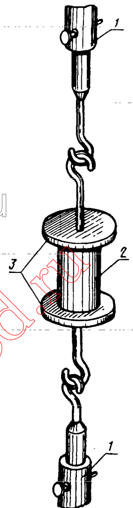
1 — зажим; 2 — образец; 3 — пластины
