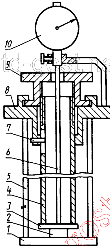
Схема прибора
