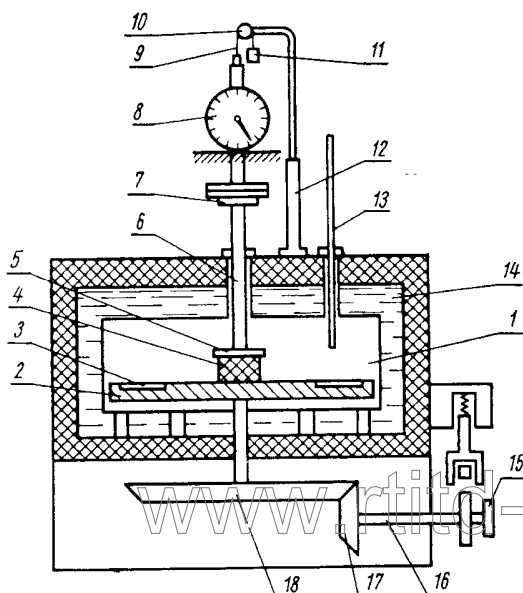
1 — испытательная камера; 2 — стол; 3 — гнезда; 4 — об-разец; 5 — мерительная площадка; 6 — шток; 7 — опорная площадка; 8 — микрометр; 9 — нить; 10 — диск; 11 — груз; 12 — стойка; 13 — термометр; 14 — емкость; 15 — рукоятка; 16 — стержень; 17 и 18 — шестерни
