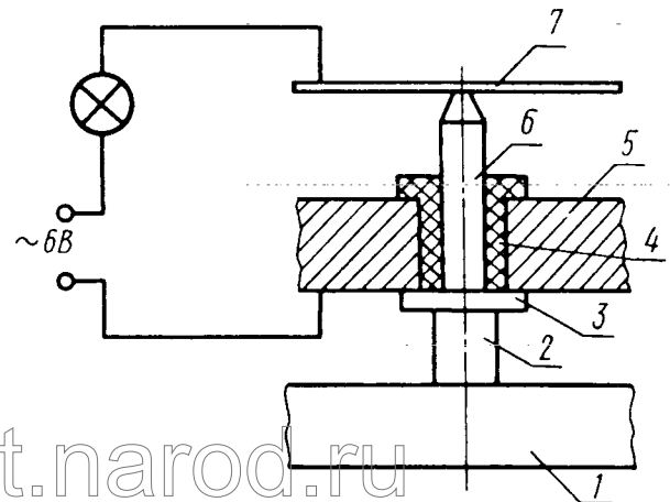
1 — нижняя плита; 2 — образец; 3 — фланец; 4 — направляющая втулка; 5 — верхняя плита; 6 — пружина; 7 — штоки
