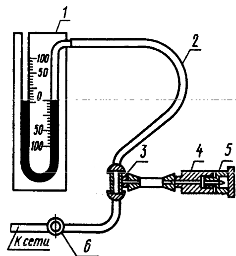
1 — ртутный манометр; 2 — шланг; 3 — тройник; 4 — патрон; 5 — пробка; 6 — кран
