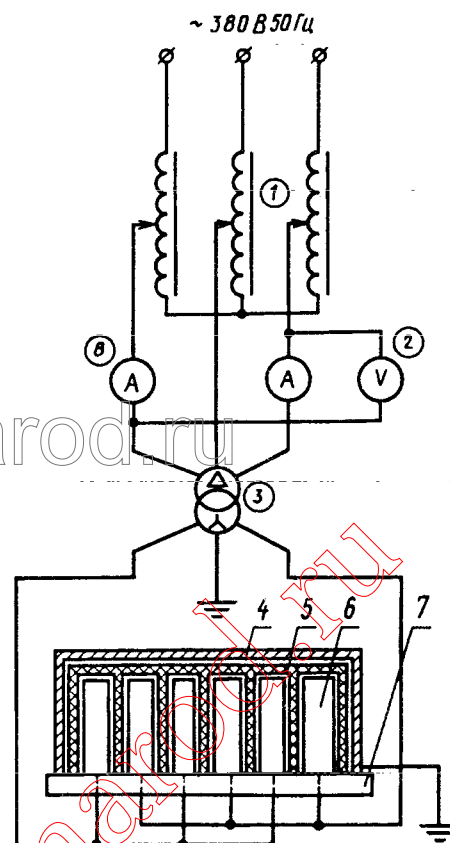
1 — автотрансформатор трехфазный регулировочный; 2 — вольтметр; 3 — трансформатор высоковольтный трехфазный; 4 — электрод корпуса моноблока; 5 — моноблок; 6 — электрод внутренний; 7 — изолирующее основание; 8 — амперметр.
