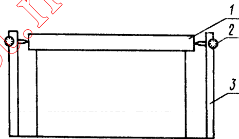
Схема замера деформации моноблока с помощью индикатора часового типа
