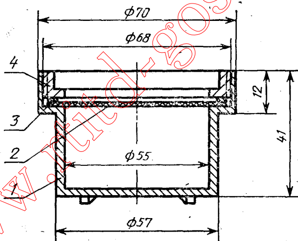
1 — стакан; 2 — образец; 3 — промежуточное кольцо; 4 — зажимная втулка
