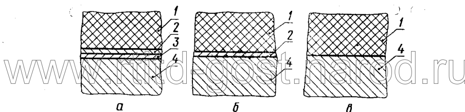
а — при применении двух клеев (методы А и В); б — при применении одного клея; в — при бесклеевом креплении (методы А и В); 1 — резина; 2 — клей; 3 — праймер; 4 — металл
