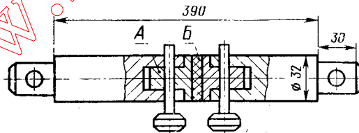
А — металлическая часть образца; Б — резина
