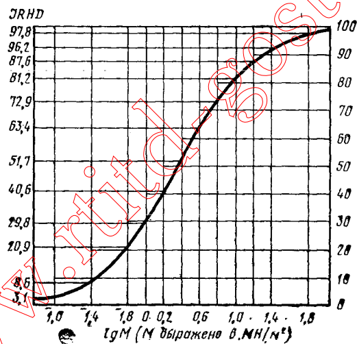
Зависимость твердости резины от модуля упругости
