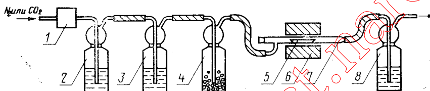
Схема установки для пиролиза
